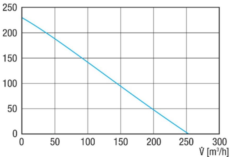
RadonTec AlphaBlower RAD 125 - Kennlinie
