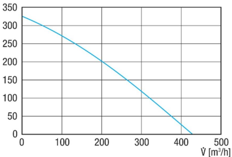
RadonTec AlphaBlower RAD 150 - Kennlinie
